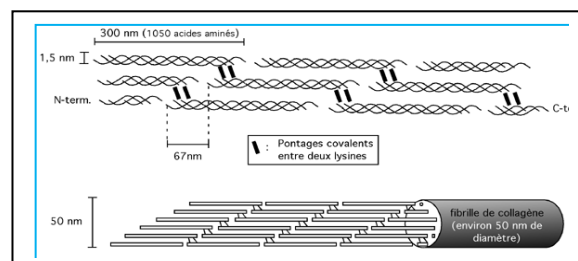
Fig.1 Le tropocollagène
